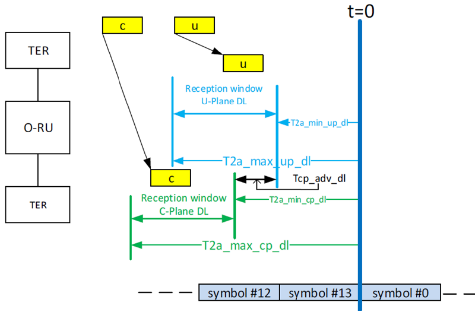
圖 15 下鏈之簡化時序
