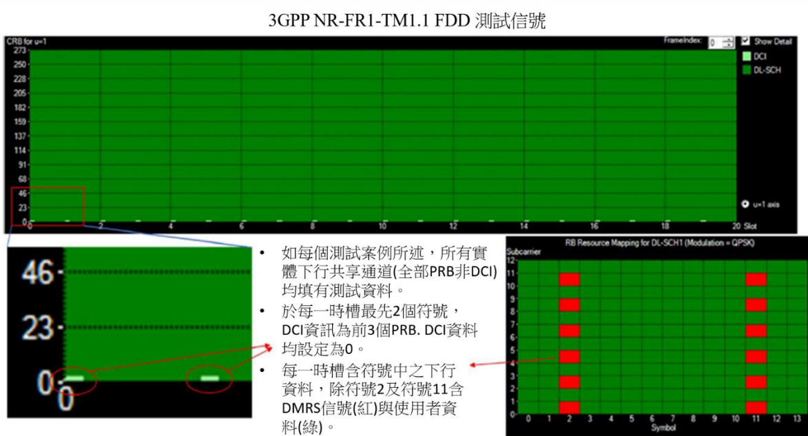
圖 9 NR-FR1-TM1.1 FDD/TDD 測試信號
