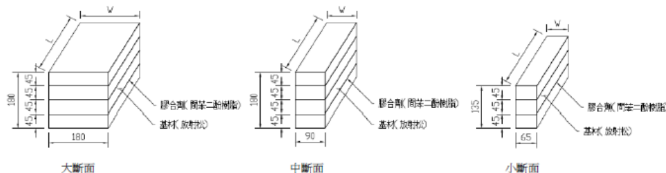
結構用集成材斷面示意圖 Unit:mm
