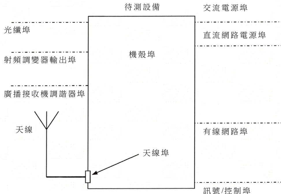
圖1 埠之範例
