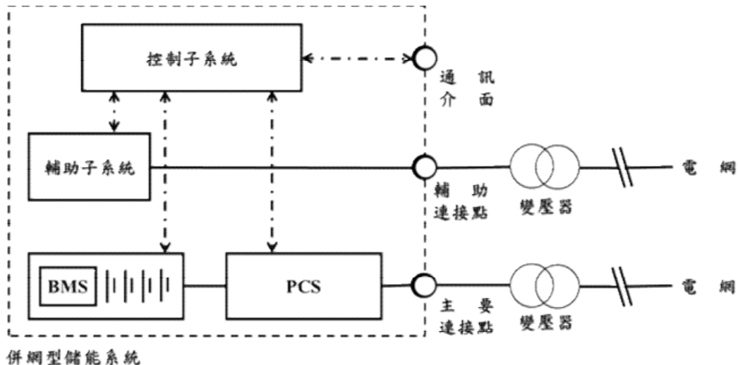
圖1 本技術規範適用範圍(併網型儲能系統為虛線範圍內)
