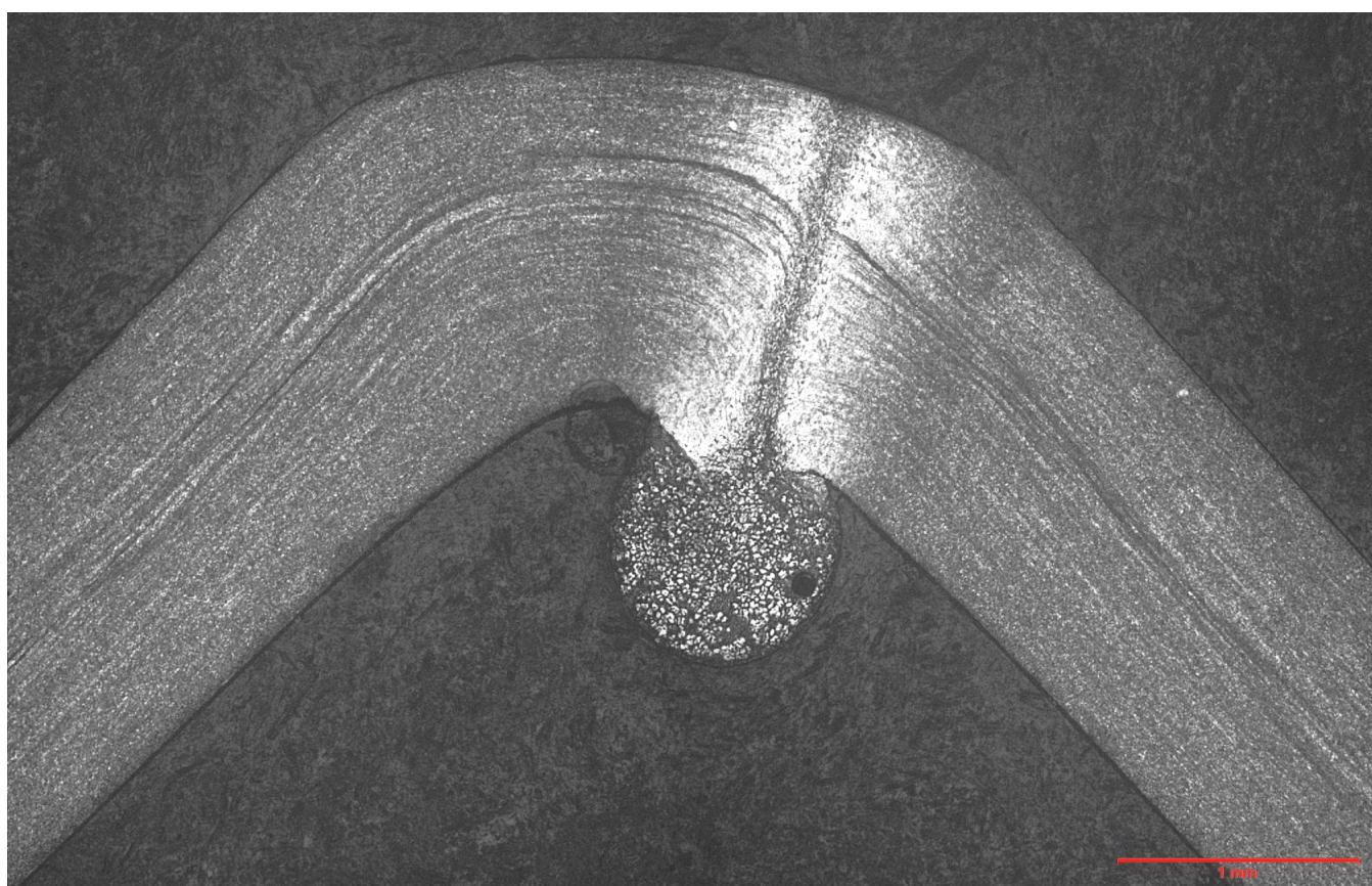
試片 2--擠壓流線圖(放大 50 倍)
