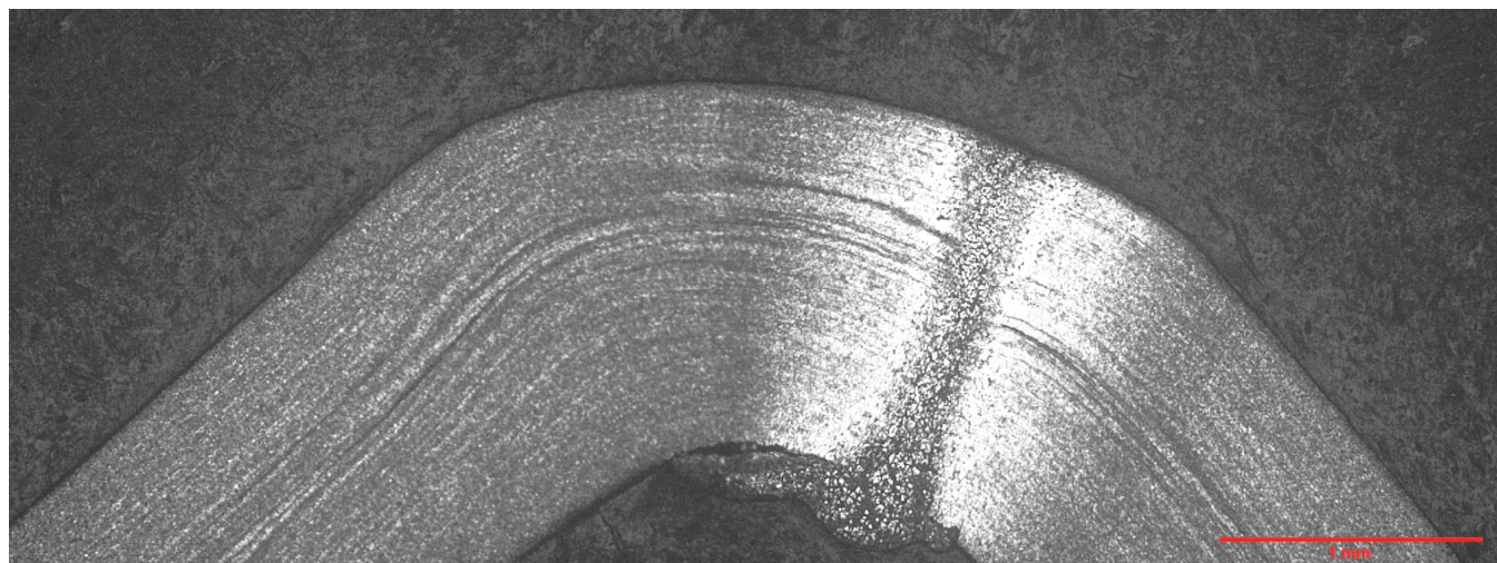
試片 1--擠壓流線圖(放大 50 倍)
