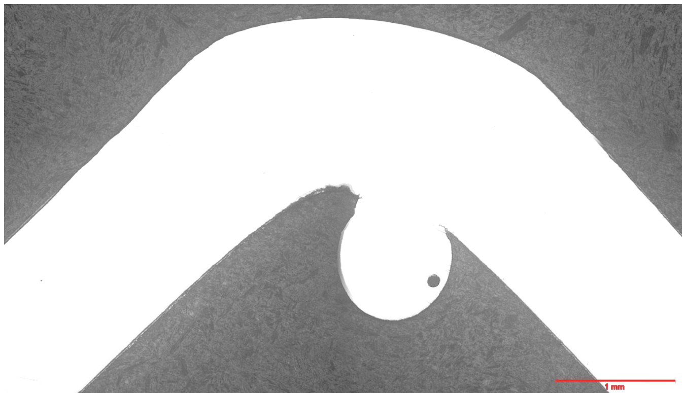
試片 2--擠壓流線圖(放大 50 倍)
