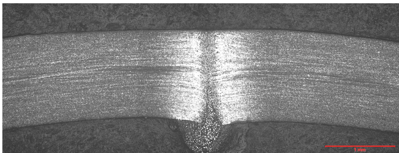
試片 3--擠壓流線圖(放大 50 倍)
