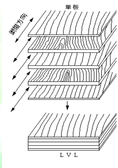
標準 層積材(角材)
