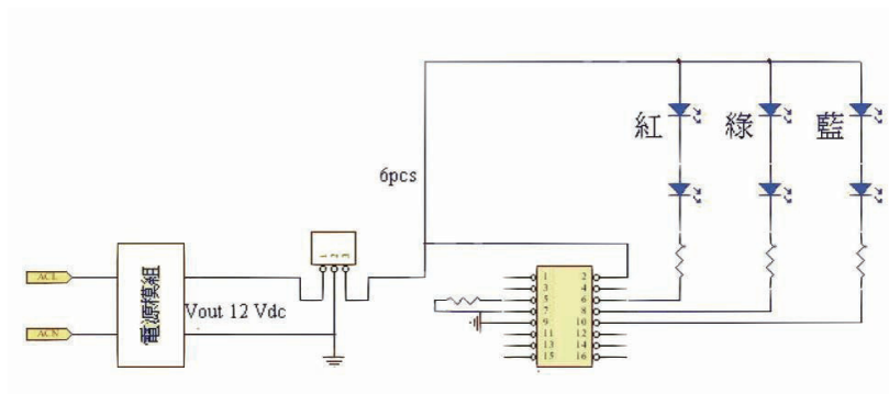
圖 4 LED 神明燈驅動電路架構 (此 IC 可驅動 6 顆 LED)
