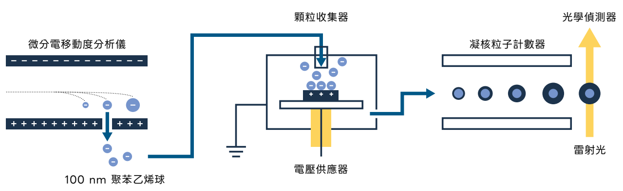
奈米粒子收集系統示意圖 ▲
