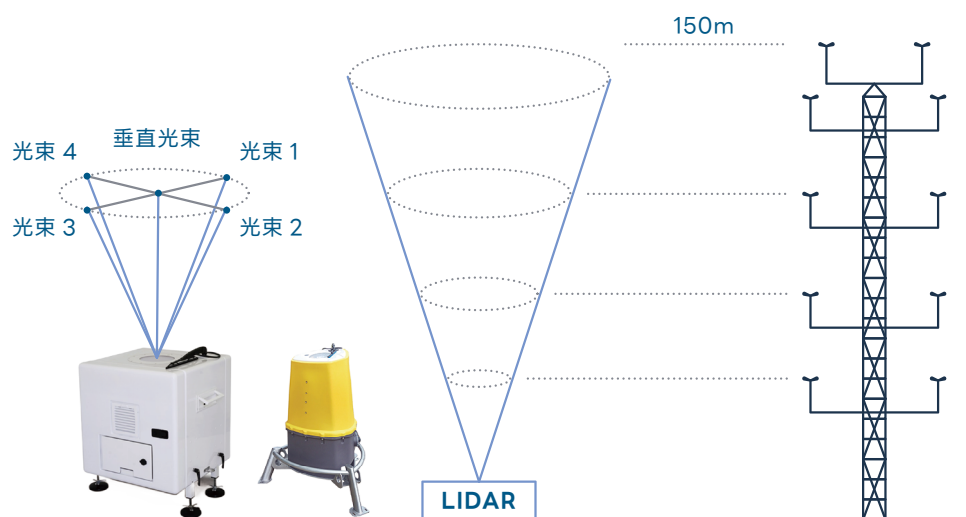
▲ 光達比對校驗示意圖
