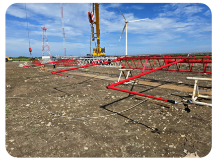
▲ 地面預組裝－ 組立儀器支架與測風儀器
