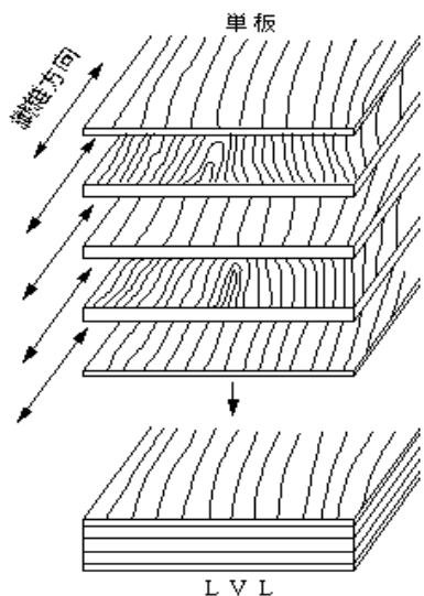
標準 層積材(角材)
